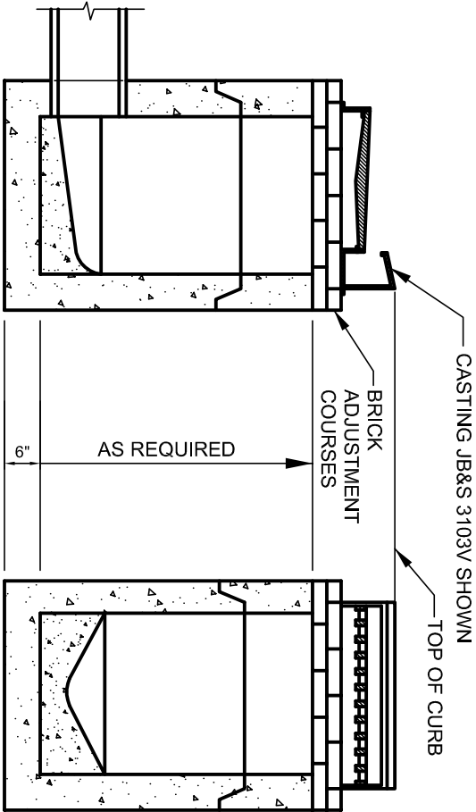
SECTION A-A
